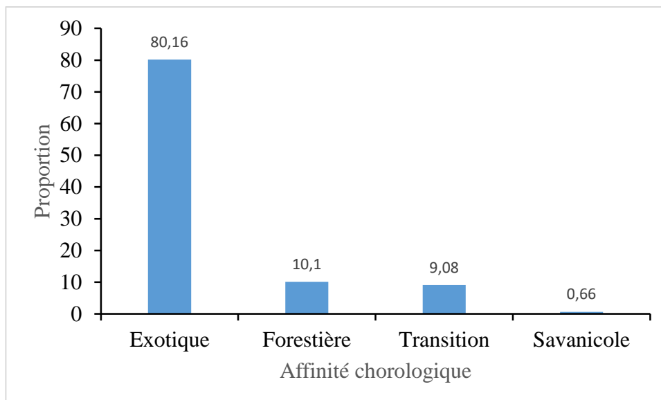
Figure 9 : Distribution de l'affinité chorologique des espèces inventoriées
